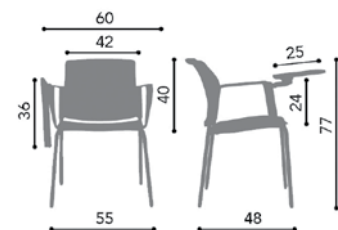
Profundidad con la pala extendida: 85 cm Profundidad con la pala en posición uso: 72 cm
